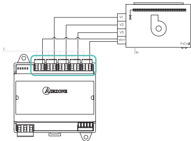
Anlage mit 2-Rohrsystem
