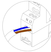
Alimentación monofásica
