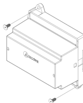
Montage mural
