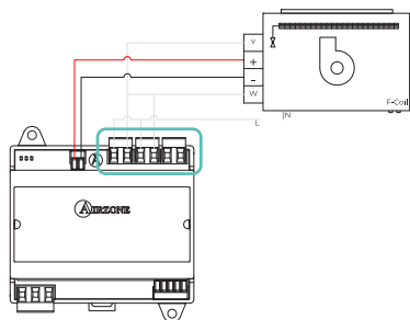
Instalacja 4-rurowa
