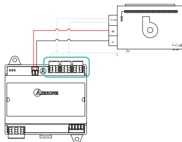
Instalacja 2-rurowa
