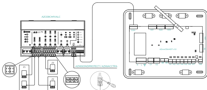
AZCE8CBIMOT pagrindinės valdymo plokštės prijungimas
