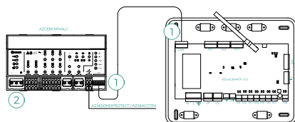
AZCE8CB1MOT pagrindinės valdymo plokštės prijungimas
