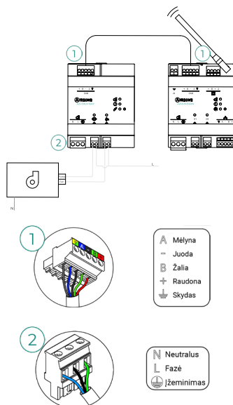
AZCE8CB1DIN pagrindinės valdymo plokštės prijungimas
