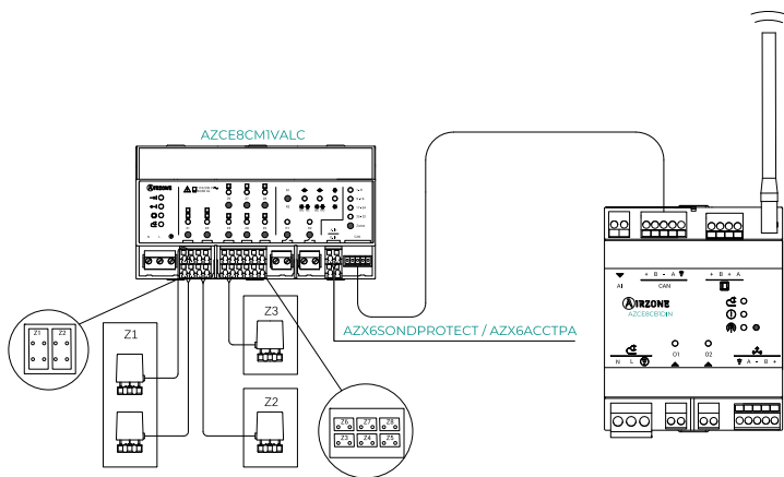
AZCE8CB1DIN pagrindinės valdymo plokštės prijungimas
