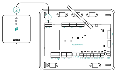
AZCE8CB1MOT pagrindinės valdymo plokštės prijungimas
