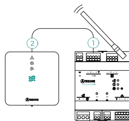
AZCE8CB1DIN pagrindinės valdymo plokštės prijungimas
