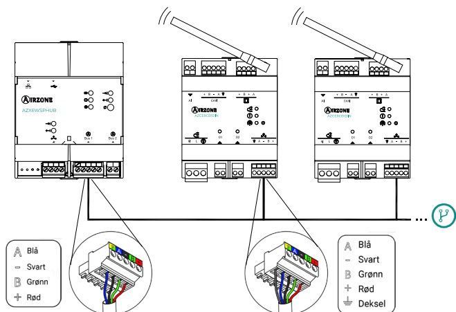
AZX6WSPHUB fra et systemhovedkontrollkort til andre systemhovedkontrollkort (AZCE8CB1DIN)
