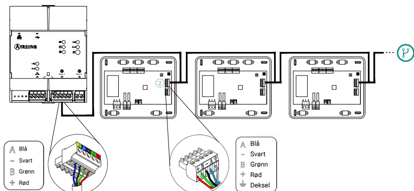
AZX6WSPHUB fra et systemhovedkontrollkort til andre systemhovedkontrollkort (AZCE8CB1MOT)
