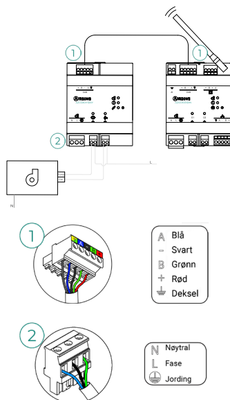
Tilkobling av hovedkontrollkortet AZCE8CB1DIN
