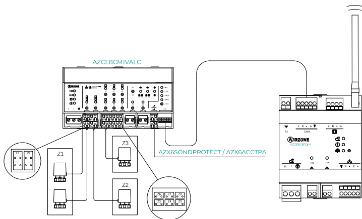
Tilkobling av hovedkontrollkortet AZCE8CB1DIN
