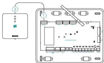
AZCE8CB1MOT tilkobling av hovedkontrollkort
