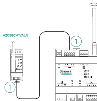
Tilkobling av hovedkontrollkortet AZCE8CB1DIN
