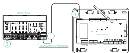
AZCE8CB1MOT tilkobling av hovedkontrollkort
