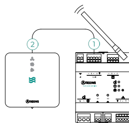
Tilkobling av hovedkontrollkortet AZCE8CB1DIN
