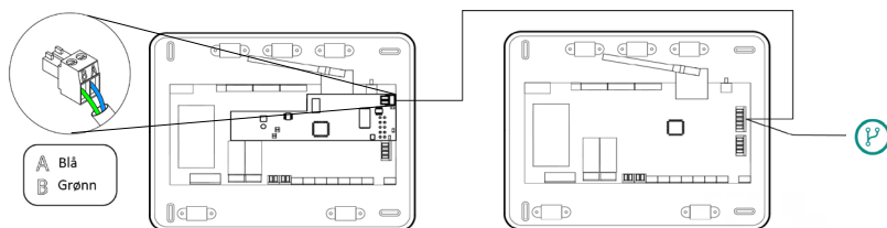
AZX6WSC5GER fra et systemhovedkontrollkort til andre systemhovedkontrollkort (AZCE8CB1MOT)
