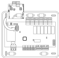
Anschluss Gateway AZX6GAW an AZX6CCPGAW
