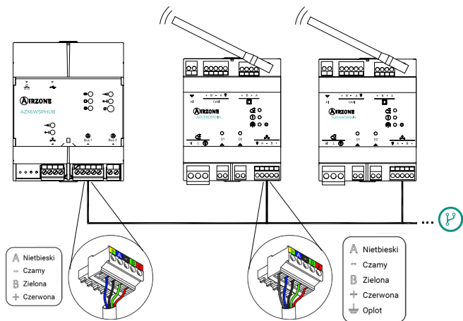
AZX6WSPHUB z centrali systemu do innych centrali systemu (AZCE8CB1DIN)
