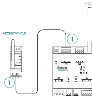
Połączenie z centralą AZCE8CB1DIN
