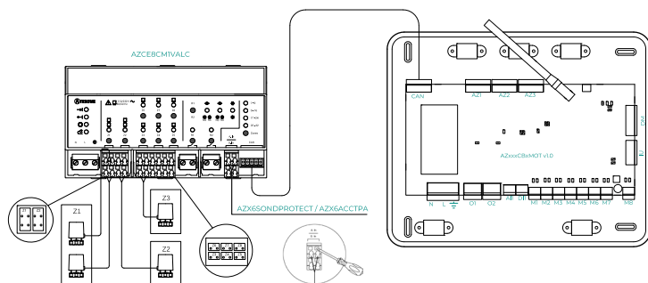
Połączenie z centralą AZCE8CB1MOT
