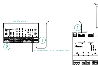
Połączenie z centralą AZCE8CB1DIN
