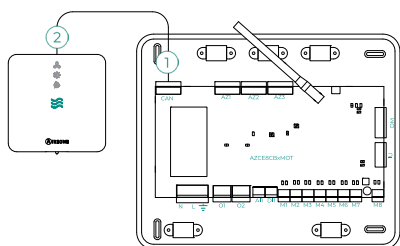
Połączenie z centralą AZCE8CB1MOT
