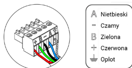
Połączenie z centralą AZCE8CB1MOT
