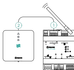
Połączenie z centralą AZCE8CB1DIN
