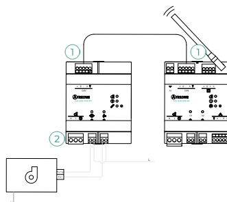
Połączenie z centralą AZCE8CB1DIN
