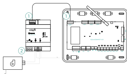
Połączenie z centralą AZCE8CB1MOT
