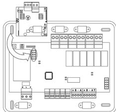
Połączenie bramy AZX8GAW / AZX6GAW z AZX6CCPGAWI
