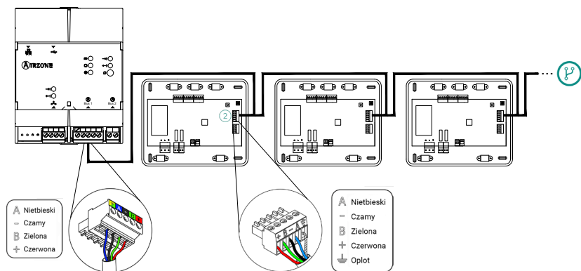
AZX6WSPHUB z centrali systemu do innych centrali systemu (AZCE8CB1MOT)
