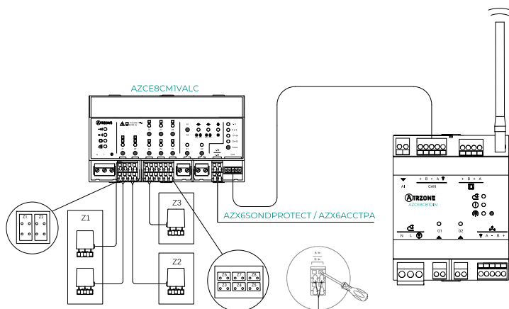
Połączenie z centralą AZCE8CB1DIN
