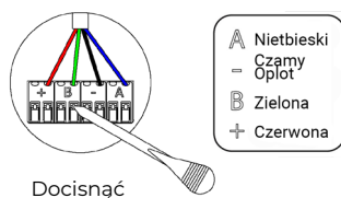
Połączenie z centralą AZCE8CB1DIN
