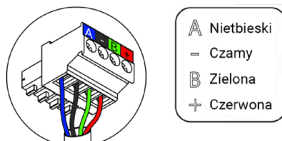
Połączenie z centralą AZCE8CB1DIN
