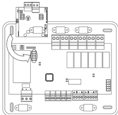
Tinklo sąsajos AZX8GAW / AZX6GAW prijungimas prie AZX6CCPGAW
