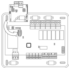
Tilkobling av gateway-AZX8GAW / AZX6GAW til AZX6CCPGAWI
