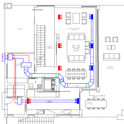
Proposta impiantistica in pianta.
