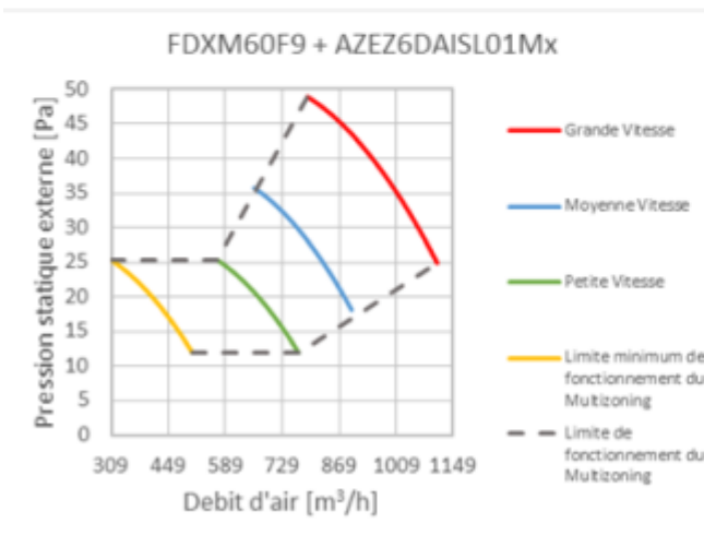
Figure 15 – Unité intérieure FDXM60F9 Courbes débit/pression
