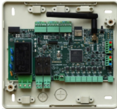
Figure 4a – Contrôleur central - AZCE8CB1MOT
