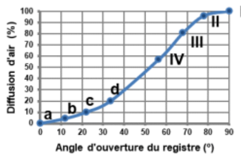
Figure 6 – Rapport entre la position d'angle d'ouverture du registre et la diffusion d'air n
