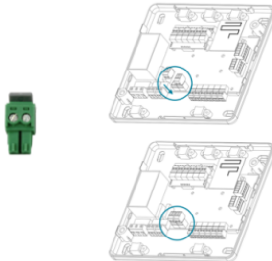
Figure 7 – Schéma d'inhibition de la fonction rafraichissement via l'accessoire AZX6MCS
