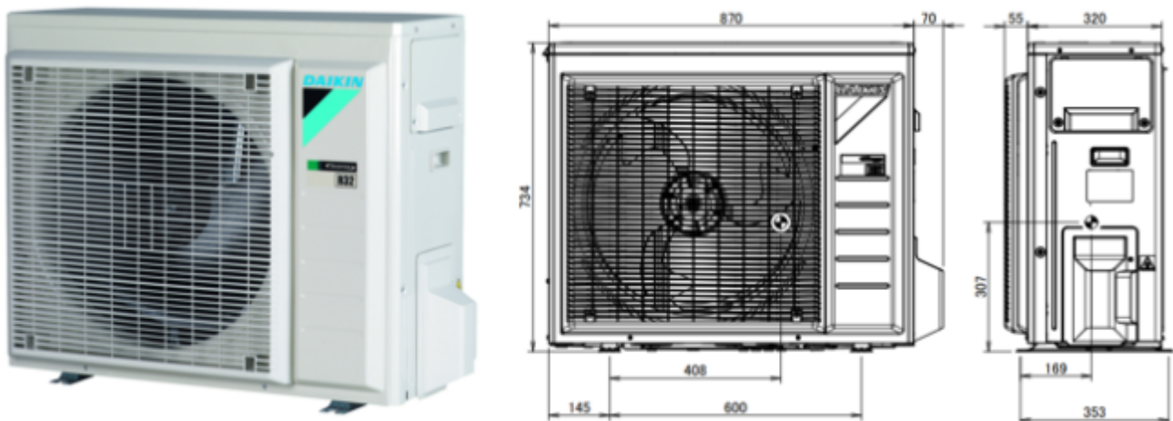
Figure 2 – Unités extérieures thermodynamiques RXM50R – visuel et caractéristiques dimensionnelles
