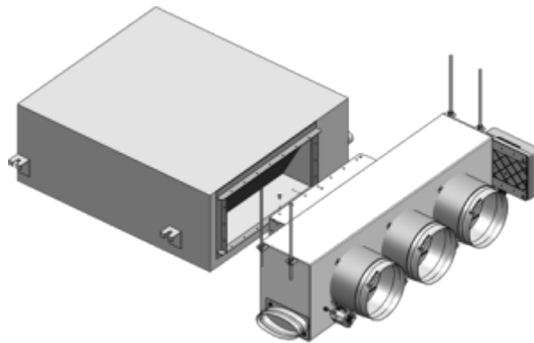
Figure 4 – Mise en œuvre du système à l'aide de pattes au plafond si besoin
