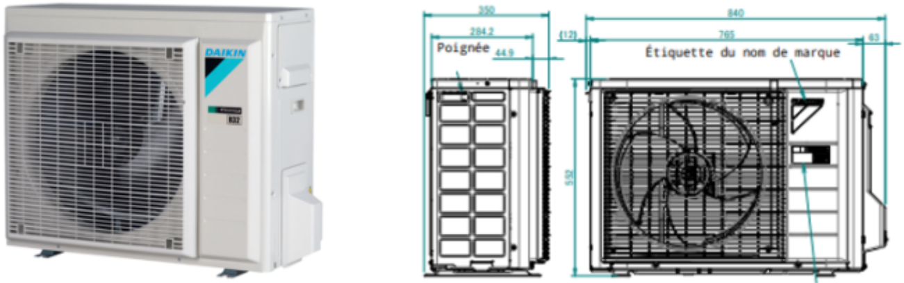
Figure 1 – Unité extérieure thermodynamique RXM35R9 – visuel et caractéristiques dimensionnelles
