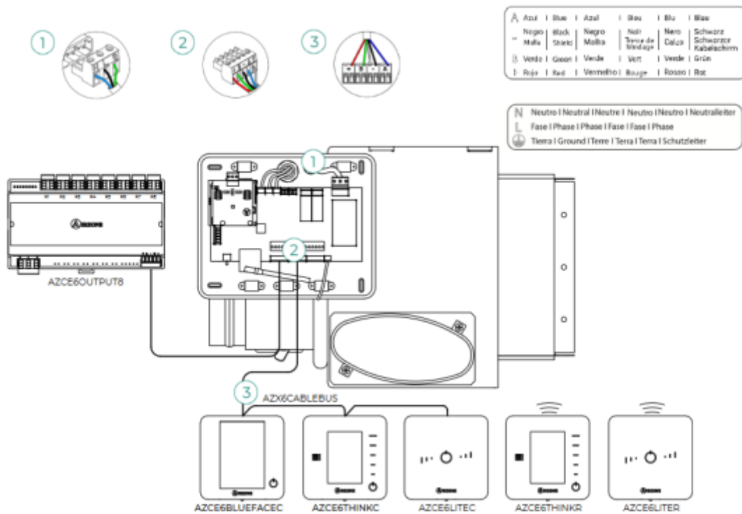
Figure 6 – Schéma d'exemple d'installation n°2
