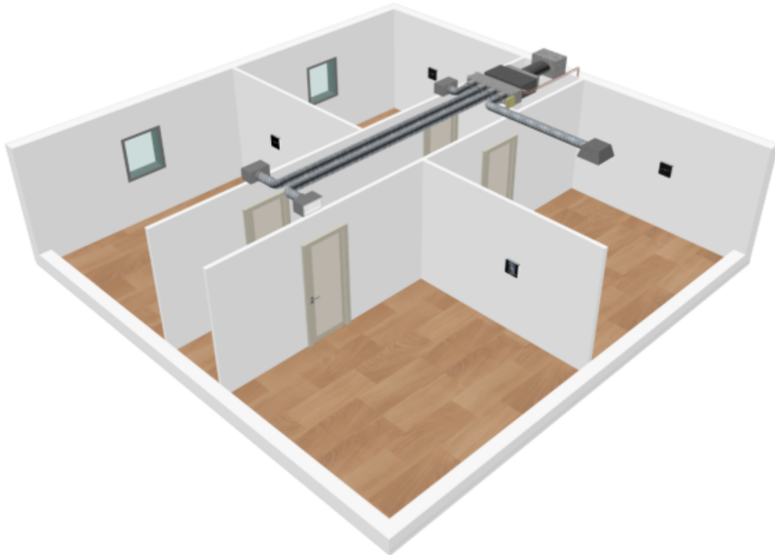
Figure 1 – Schéma de principe du système « Gainable Daikin et Multizoning Airzone »
