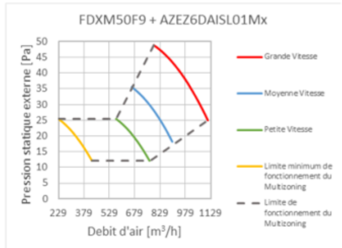
Figure 14 – Unité intérieure FDXM50F9 Courbes débit/pression
